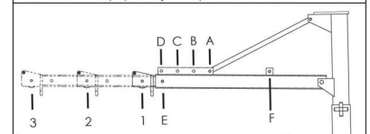
BOOM CAPACITY CHART: WTJ-E-15-3 (AC or DC) Tabla de capacidad del auge: WTJ-E-15-3
